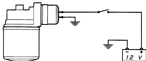
SCHEMA ELETTRICO
